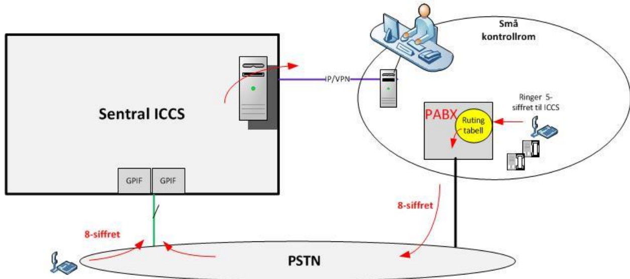
Fig 2: Omrouting av telefonsamtaler I PABX
