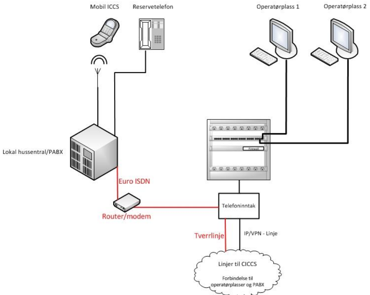
Fig 1 Rød linje viser tverrlinjen mellom CICCS og PABX
